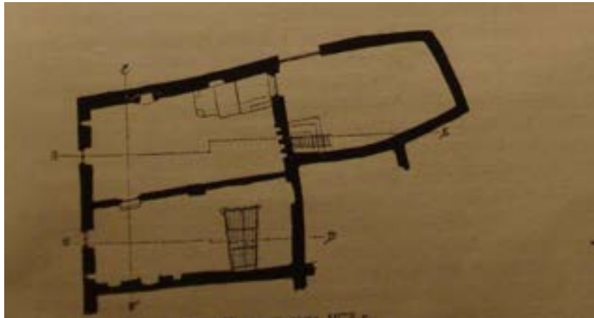
асад дома 1 7 г.в ауле Корода о обмеру с натуры 19 г.
