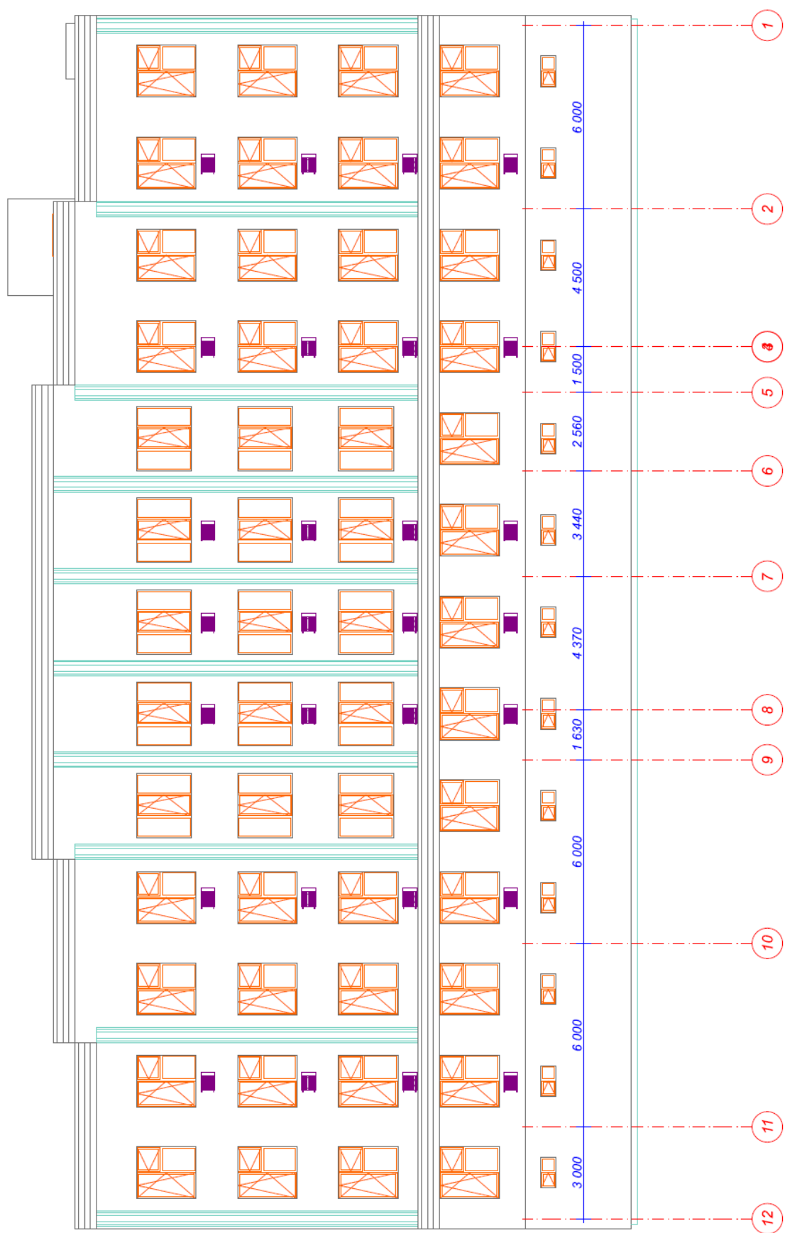
Илл. 8. Фасад в осях 12-1
