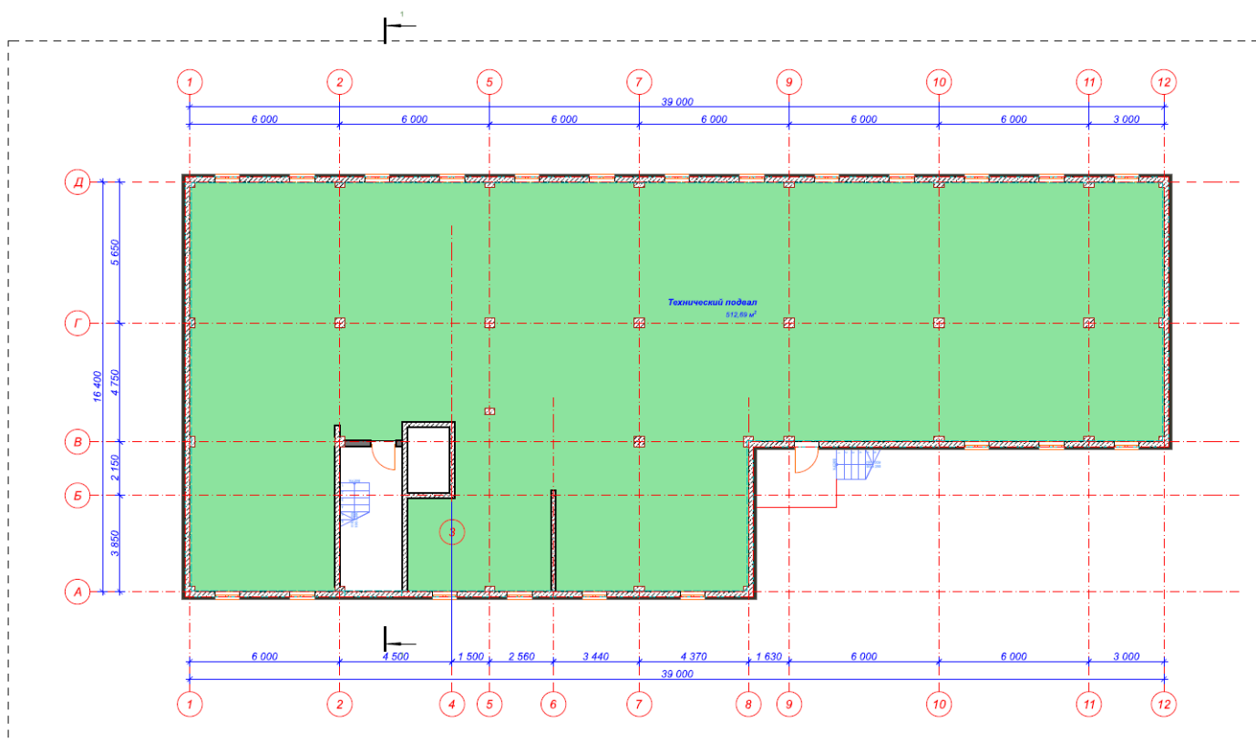
Илл.3. План подвального этажа
