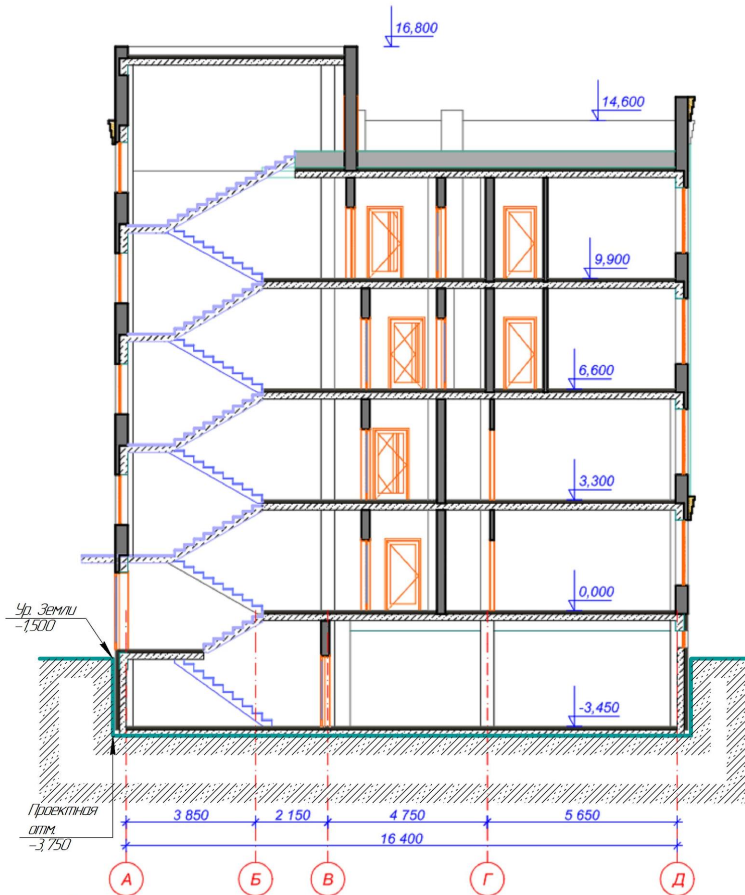
Илл. 10. Разрез 1-1
