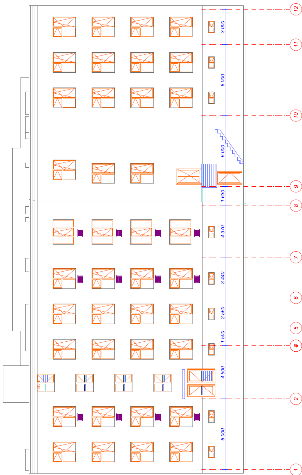
Илл. 9. Фасад в осях 1-12
