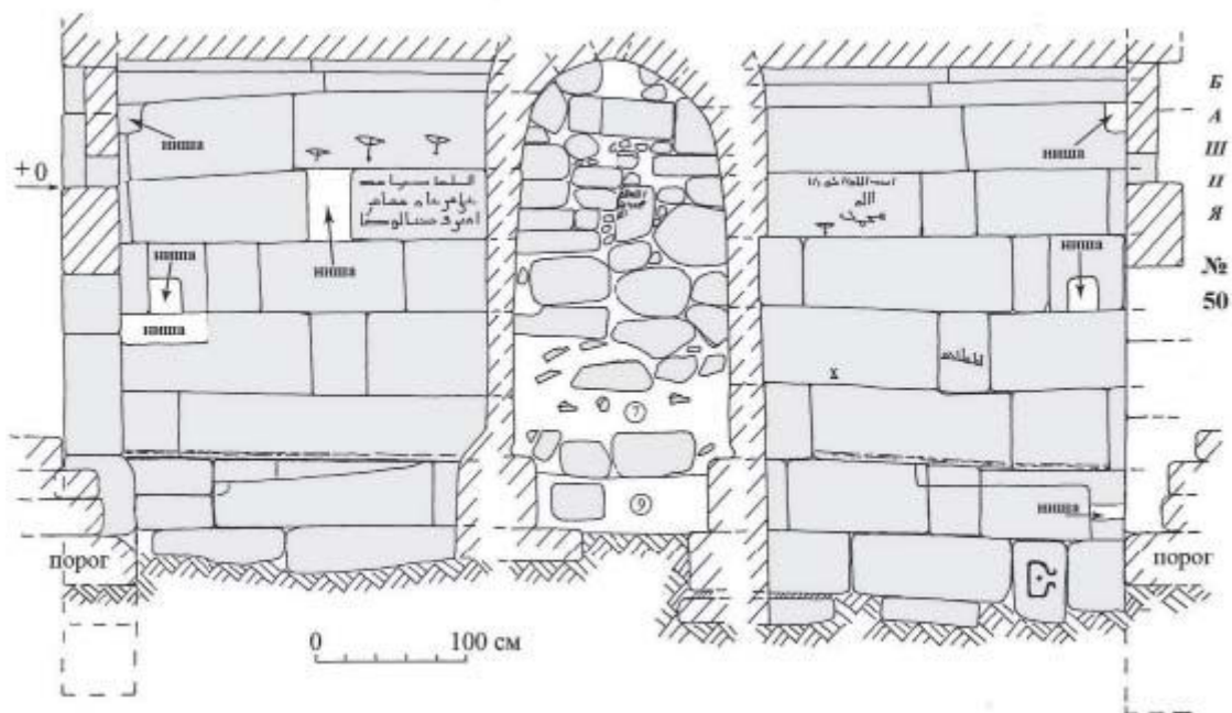
Илл. 15. Дербент. Культовое место Баб ал-Кийама. Разверстка стен арочного прохода
