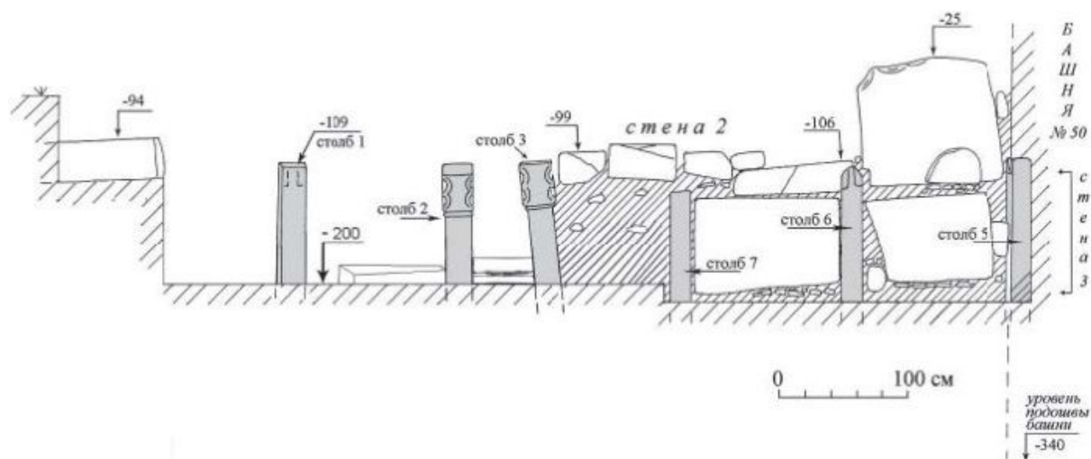
Илл. 10. Дербент. Культовое место Баб ал-Кийама. Профиль стены ограды и прохода с резными столбами
