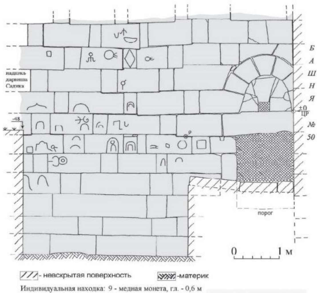
Илл. 14. Дербент. Культовое место Баб ал-Кийама. Профиль оборонительной стены с арочным проходом со смотровым окном около баини 50
