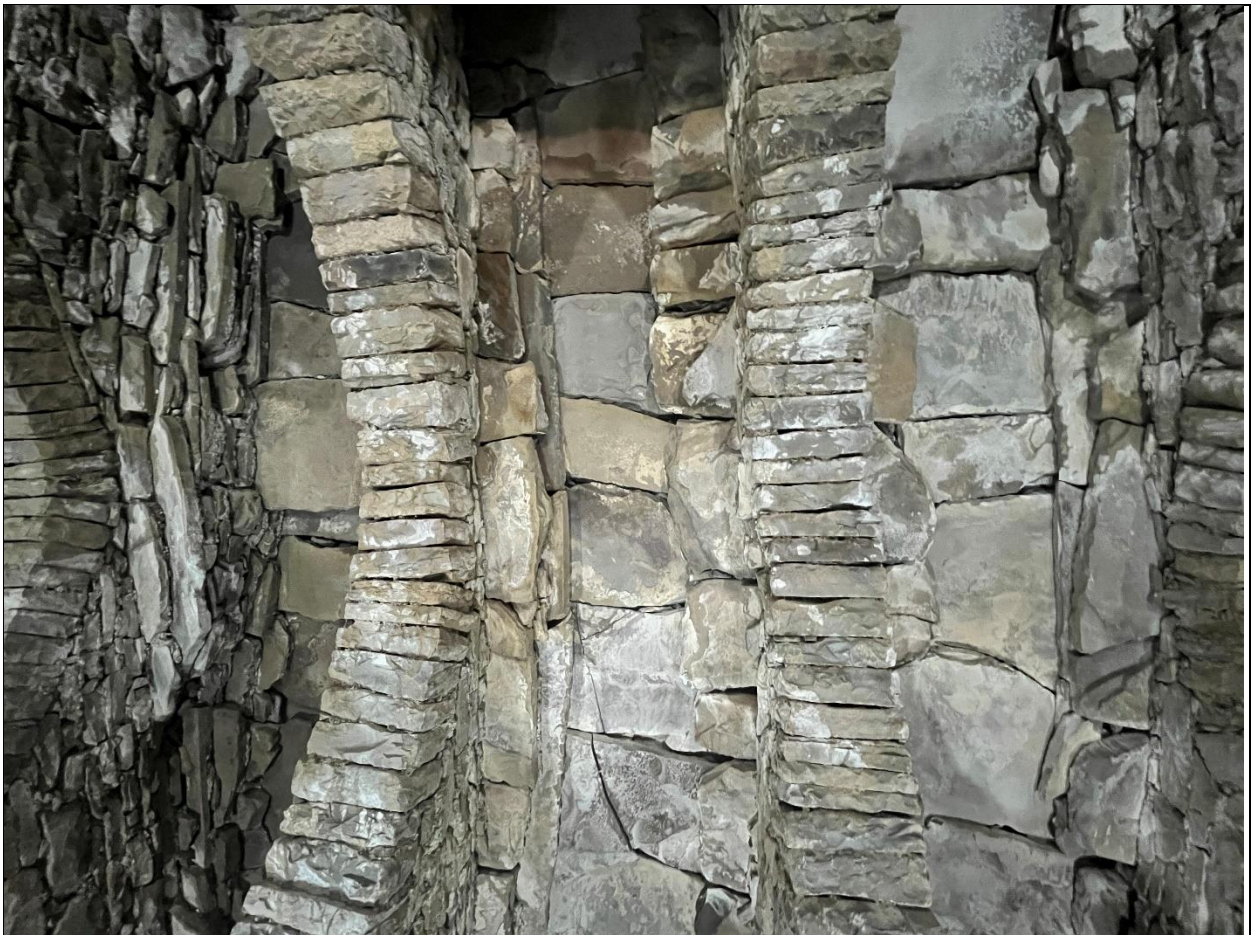
Фото 3. Сводчатое перекрытие мечети
