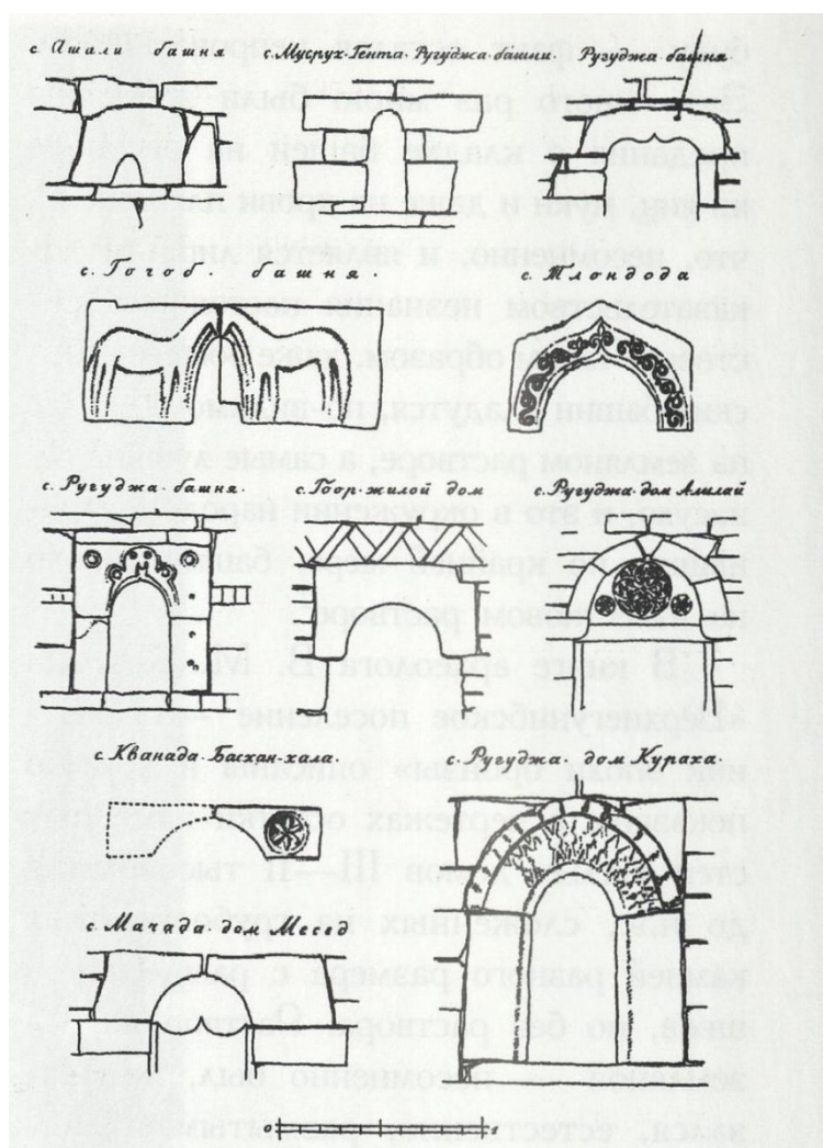
Илл. 3. Таблица архаических каменных арок до знакомства с клинчатой конструкцией
