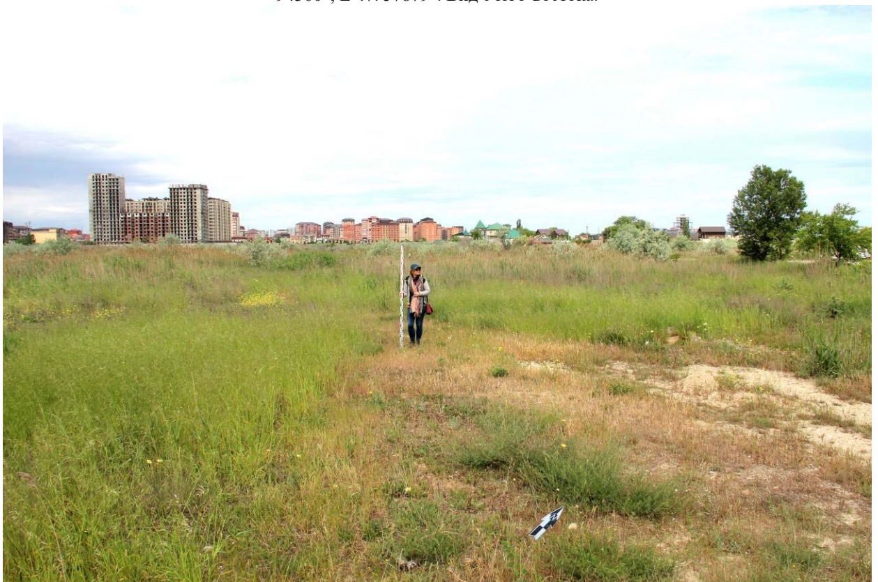
Рис. 57. Республика Дагестан. Объект «Проектирование и строительство напорной нитки D 1400 мм от ГКНС-6 г. Махачкалы до канализационных очистных сооружений г. Каспийска протяжённостью 16,0 км и производительностью 300 тыс. куб. м. в сутки». Трасса обследования. Точка фиксации №30 (WGS-84) N 42.94658°; E 47.57609°. Вид с юго-востока.
