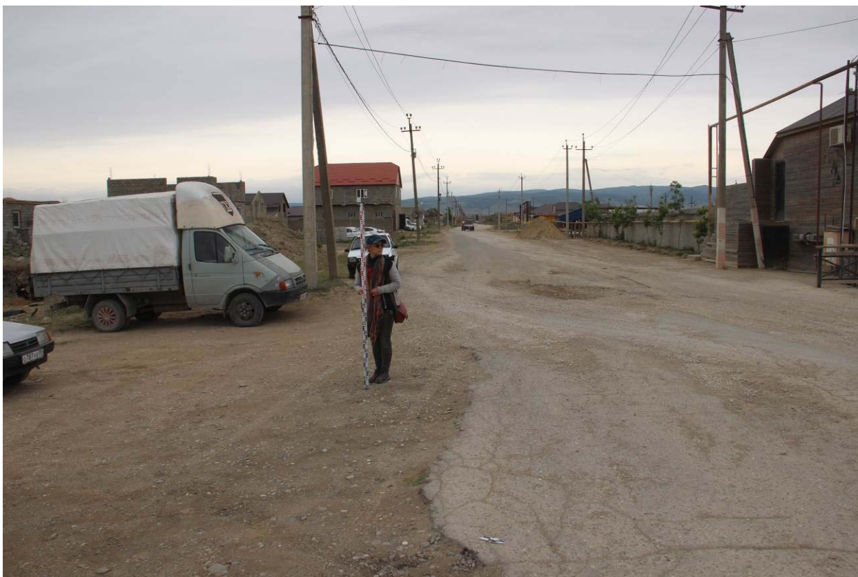
Рис.4. Республика Дагестан. Объект «Проектирование и строительство напорной нитки D 1400 мм от ГКНС-6 г. Махачкалы до канализационных очистных сооружений г. Каспийска протяжённостью 16,0 км и производительностью 300 тыс. куб. м. в сутки». Трасса обследования. Точка фиксации №1 (WGS-84) N 42.86723°; E 47.67640°. Улица Маячная 129 (1-я Карьерная линия). Вид с востока.
