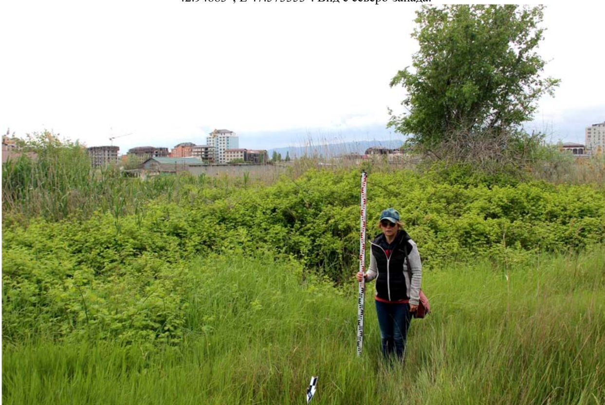
Рис. 61. Республика Дагестан. Объект «Проектирование и строительство напорной нитки D 1400 мм от ГКНС-6 г. Махачкалы до канализационных очистных сооружений г. Каспийска протяжённостью 16,0 км и производительностью 300 тыс. куб. м. в сутки». Трасса обследования. Точка фиксации №32 (WGS-84) N 42.950224°; E 47.573106°. Вид с севера.
