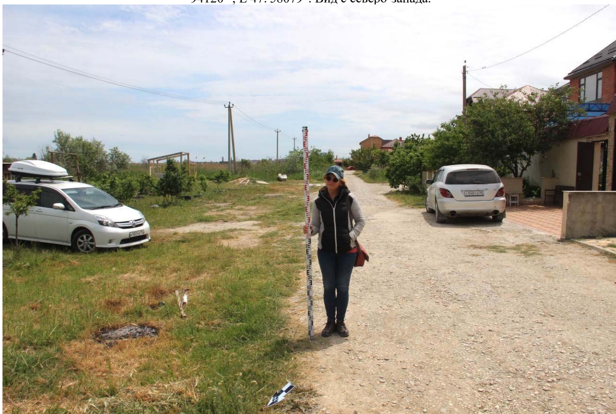
Рис. 55. Республика Дагестан. Объект «Проектирование и строительство напорной нитки D 1400 мм от ГКНС-6 г. Махачкалы до канализационных очистных сооружений г. Каспийска протяжённостью 16,0 км и производительностью 300 тыс. куб. м. в сутки». Трасса обследования. Точка фиксации №29 (WGS-84) N 42. 94360°; E 47. 57879°. Вид с северо-запада.
