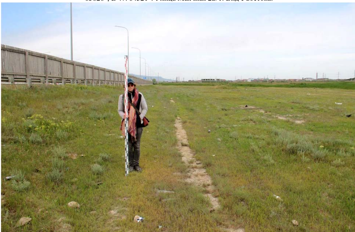
Рис. 17. Республика Дагестан. Объект «Проектирование и строительство напорной нитки D 1400 мм от ГКНС-6 г. Махачкалы до канализационных очистных сооружений г. Каспийска протяжённостью 16,0 км и производительностью 300 тыс. куб. м. в сутки». Трасса обследования. Точка фиксации №8 (WGS-84) N 42. 857353°; E 47. 639733°. Вид с юго-востока.
