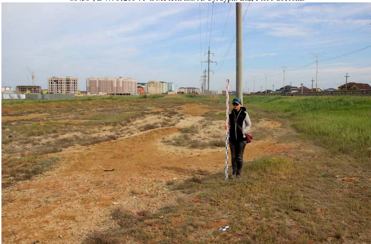
Рис. 35. Республика Дагестан. Объект «Проектирование и строительство напорной нитки D 1400 мм от ГКНС-6 г. Махачкалы до канализационных очистных сооружений г. Каспийска протяжённостью 16,0 км и производительностью 300 тыс. куб. м. в сутки». Трасса обследования. Точка фиксации №18 (WGS-84) N 42. 88863°; E 47. 60437°. Вид с северо-запада.
