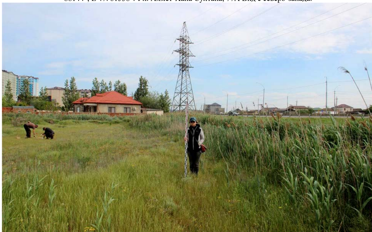
Рис. 33. Республика Дагестан. Объект «Проектирование и строительство напорной нитки D 1400 мм от ГКНС-6 г. Махачкалы до канализационных очистных сооружений г. Каспийска протяжённостью 16,0 км и производительностью 300 тыс. куб. м. в сутки». Трасса обследования. Точка фиксации №17 (WGS-84) N 42. 88458°; E 47. 61200°. Р-н Мечети им. А. Сугъури. Вид с северо-запада.
