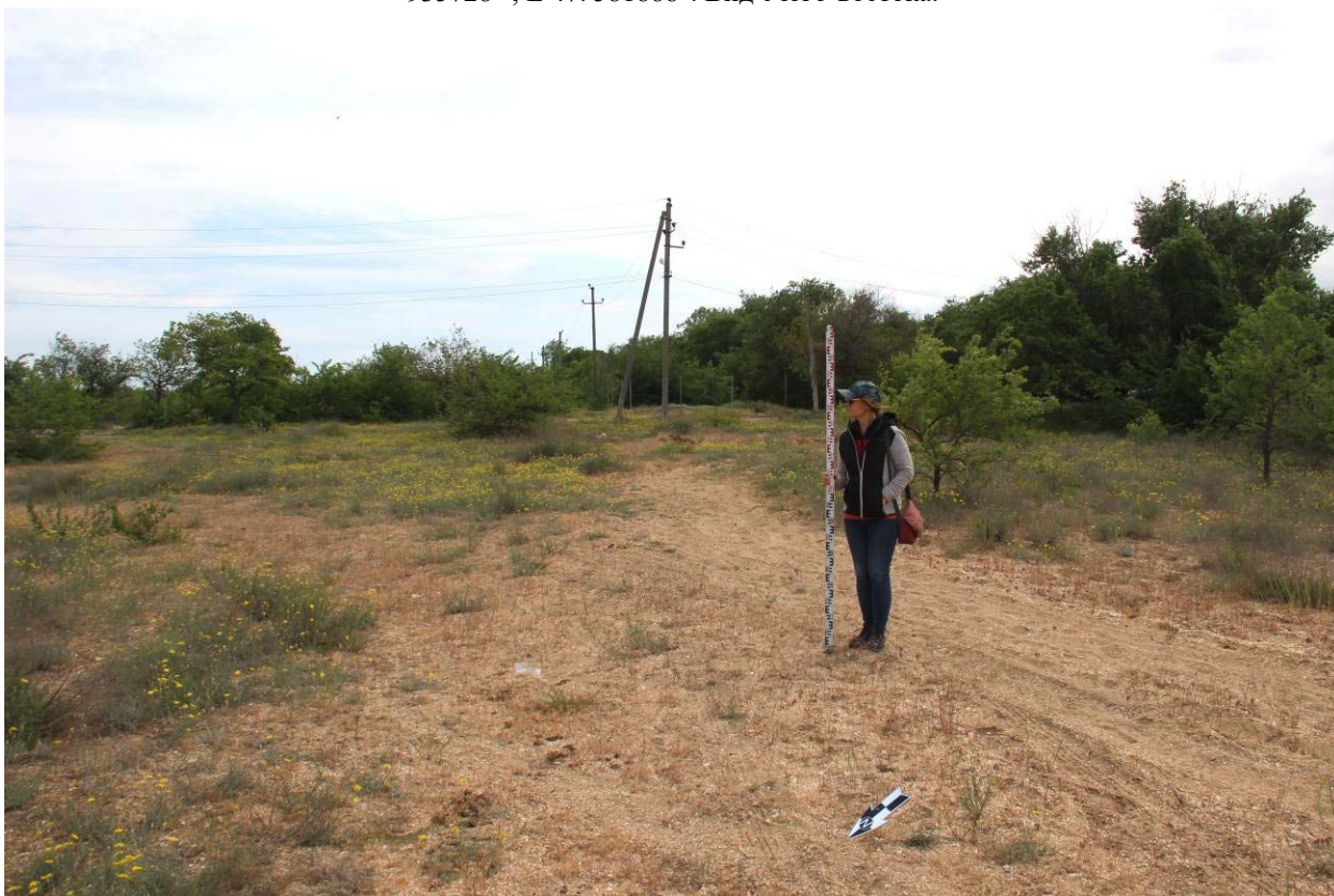
Рис. 53. Республика Дагестан. Объект «Проектирование и строительство напорной нитки D 1400 мм от ГКНС-6 г. Махачкалы до канализационных очистных сооружений г. Каспийска протяжённостью 16,0 км и производительностью 300 тыс. куб. м. в сутки». Трасса обследования. Точка фиксации №27 (WGS-84) N 42. 935728 °; E 47. 581888°. Вид с северо-запада.
