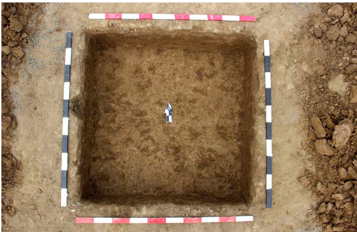
Рис. 99. Республика Дагестан. Объект «Проектирование и строительство напорной нитки D 1400 мм от ГКНС-6 г. Махачкалы до канализационных очистных сооружений г. Каспийска протяжённостью 16,0 км и производительностью 300 тыс. куб. м. в сутки». Шурф 7 после окончания земляных работ. Шурф на уровне материкового туго-пластичного суглинка светло-коричневого оттенка. Вид с юга сверху.
