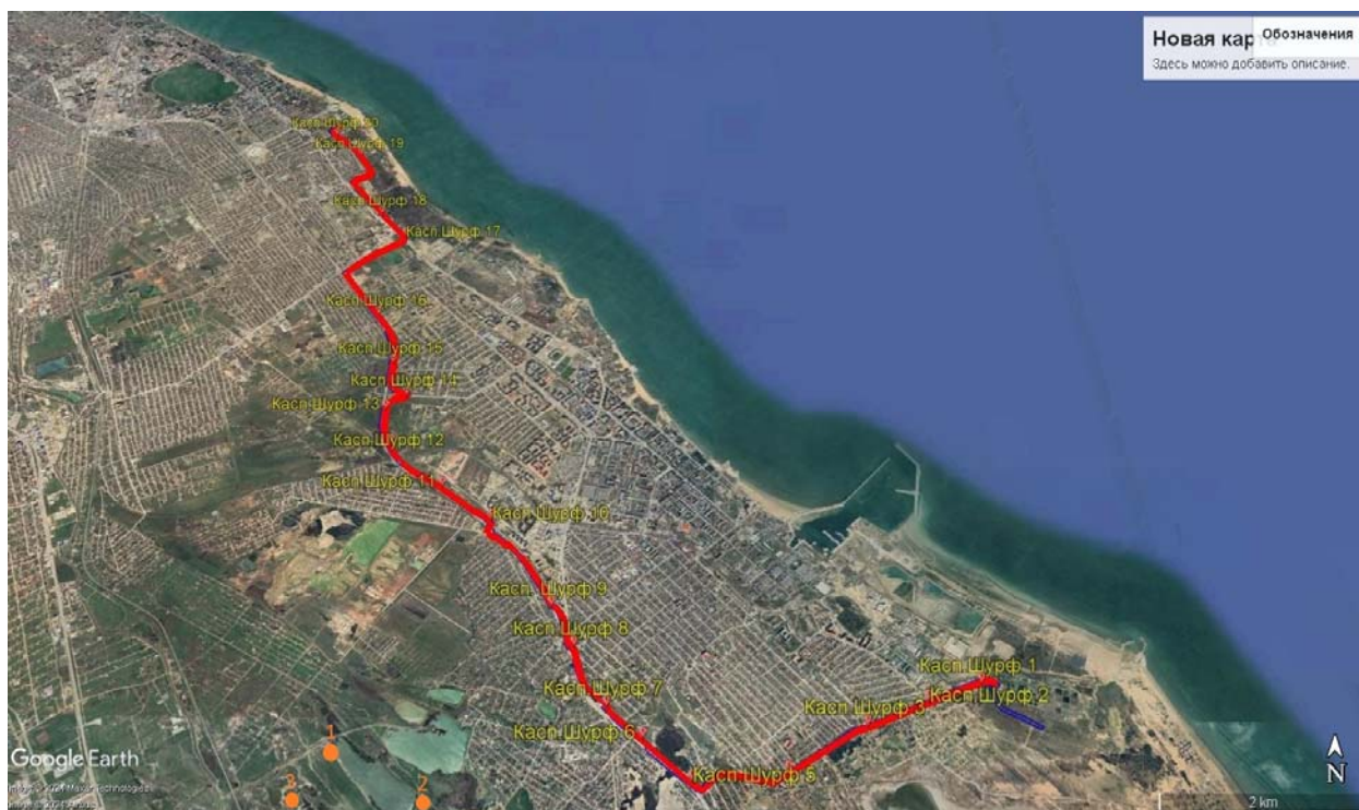
Рис. 2. Республика Дагестан. Объект «Проектирование и строительство напорной нитки D 1400 мм от ГКНС-6 г. Махачкалы до канализационных очистных сооружений г. Каспийска протяжённостью 16,0 км и производительностью 300 тыс. куб. м. в сутки» - ближайшие ОАН.
