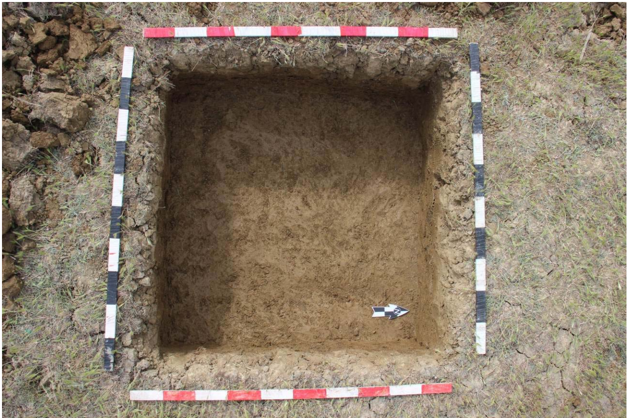
Рис. 112. Республика Дагестан. Объект «Проектирование и строительство напорной нитки D 1400 мм от ГКНС-6 г. Махачкалы до канализационных очистных сооружений г. Каспийска протяжённостью 16,0 км и производительностью 300 тыс. куб. м. в сутки». Шурф 10 после окончания земляных работ. Шурф на уровне материкового туго-пластичного суглинка светло-коричневого оттенка. Уровень выхода грунтовых вод. Вид с востока сверху.
