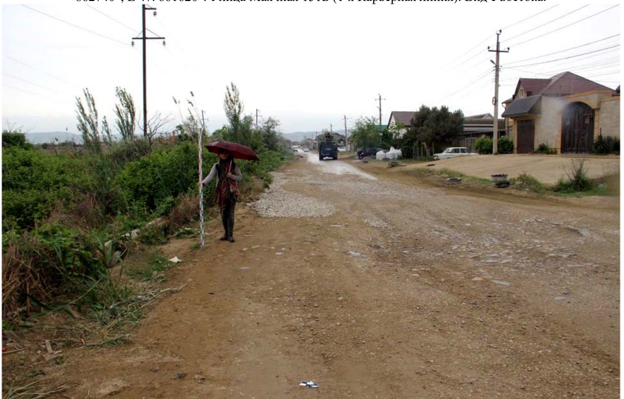
Рис. 9. Республика Дагестан. Объект «Проектирование и строительство напорной нитки D 1400 мм от ГКНС-6 г. Махачкалы до канализационных очистных сооружений г. Каспийска протяжённостью 16,0 км и производительностью 300 тыс. куб. м. в сутки». Трасса обследования. Точка фиксации №4 (WGS-84) N 42. 86215°; E 47. 65960°. Улица Маячная 151. Вид с востока.
