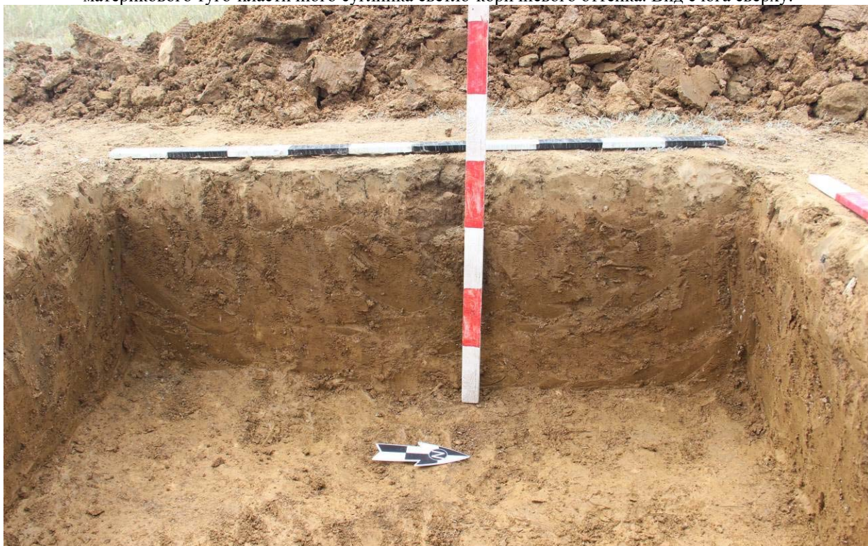
Рис. 100. Республика Дагестан. Объект «Проектирование и строительство напорной нитки D 1400 мм от ГКНС-6 г. Махачкалы до канализационных очистных сооружений г. Каспийска протяжённостью 16,0 км и производительностью 300 тыс. куб. м. в сутки». Зачистка шурфа 7 на уровне материкового туго-пластичного суглинка светло-коричневого оттенка. Стратиграфия профиля западного борта шурфа. Вид с востока.
