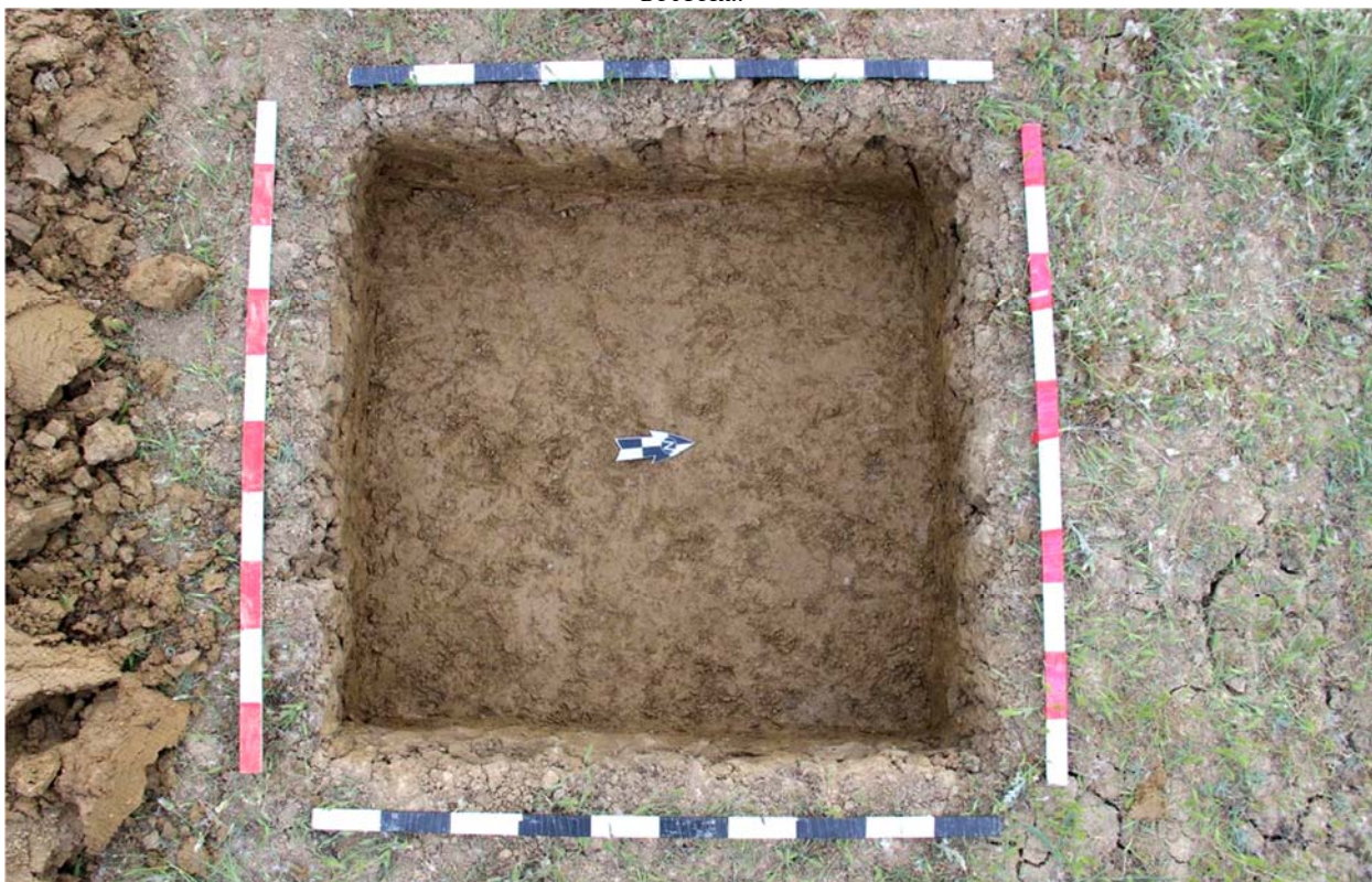
Рис. 132. Республика Дагестан. Объект «Проектирование и строительство напорной нитки D 1400 мм от ГКНС-6 г. Махачкалы до канализационных очистных сооружений г. Каспийска протяжённостью 16,0 км и производительностью 300 тыс. куб. м. в сутки». Шурф 14 после окончания земляных работ. Шурф на уровне материкового туго-пластичного суглинки светло-коричневого оттенка. Вид с востока сверху.
