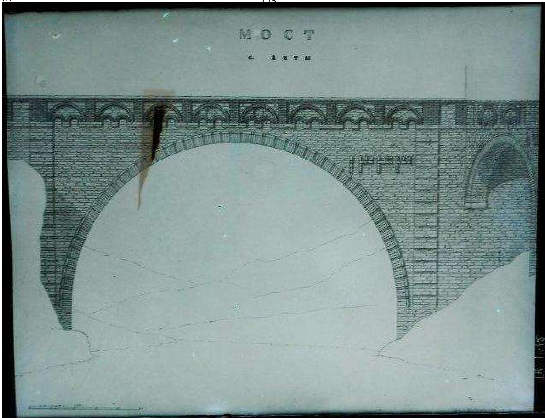
Негатив. Мост в селе Ахты. Дагестан. Обмерный чертеж. Фасад. 1940 - 1956 год //ГНИМА НФ-ОФ-984/741
